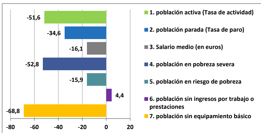
Gráfico 4. Resultados de indicadores inclusión social de la población con discapacidad. Diferencia porcentual. Eje económico.
